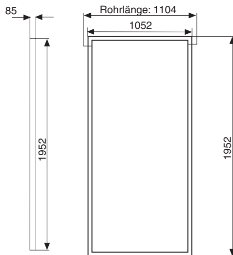
Kollektorabmessungen in mm
